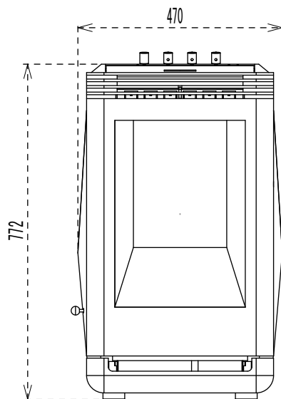
正面
