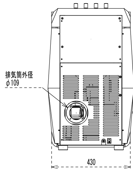
背面
