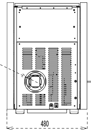
背面
