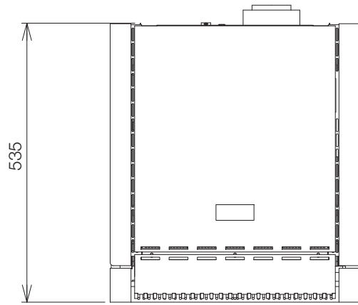
平面
